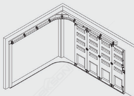
▲ Pintu Dorong Menikung Eksterior Roda "Standard"
